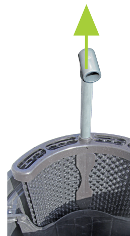
corps du préfiltre
