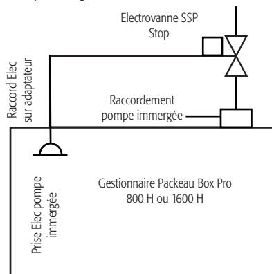
Vue arrière
